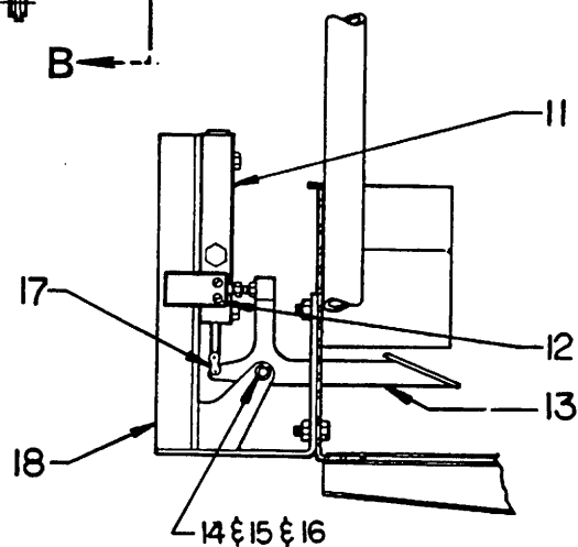
VIEW A-A
